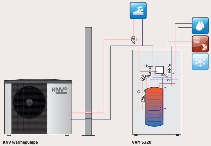
KNV Wärmepumpe
